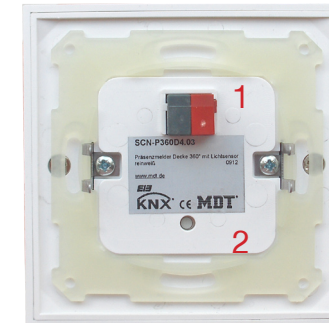
SCN-P360x3.03 Rückansicht - Back view
